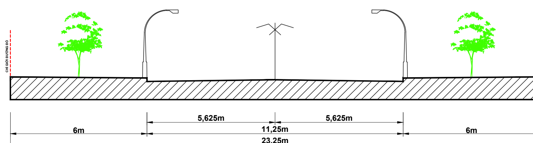
CẮT 1-1
